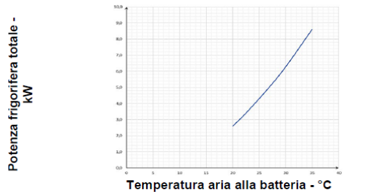
POTENZA FRIGORIFERA (4)
