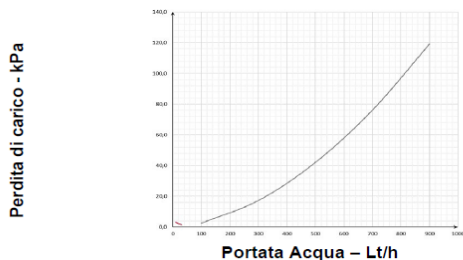
PERDITE DI CARICO/PORTATE BATTERIA IDRONICA
