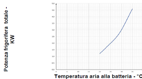
RESA FRIGORIFERA BATTERIA IDRONICA (4)
