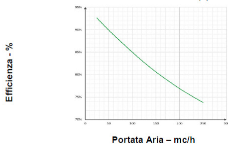
EFFICIENZA TERMICA (1)
