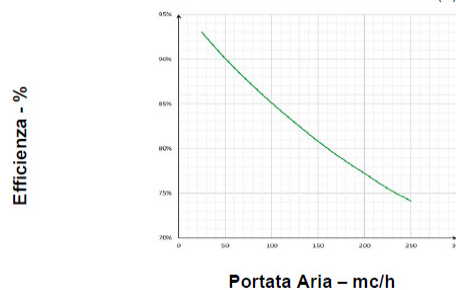
EFFICIENZA TERMICA ESTIVA (2)
