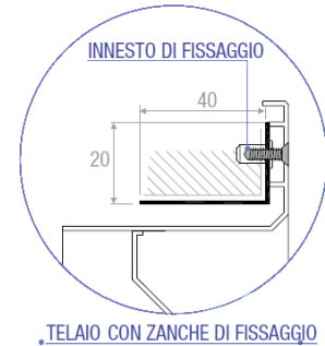
CONTROTELAIO DI FISSAGGIO
