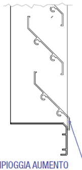
EGRIA5 + TEGOLO ANTIPIOGGIA
